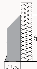
IP 30-40-50 С ВЫКРУЖКОЙ / ПРЯМОЙ
