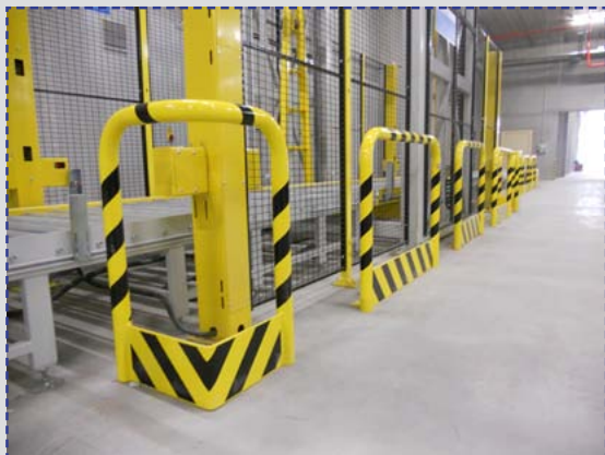
PolySto PMA (лев.) and PML (прав.) на бетонном полу.
