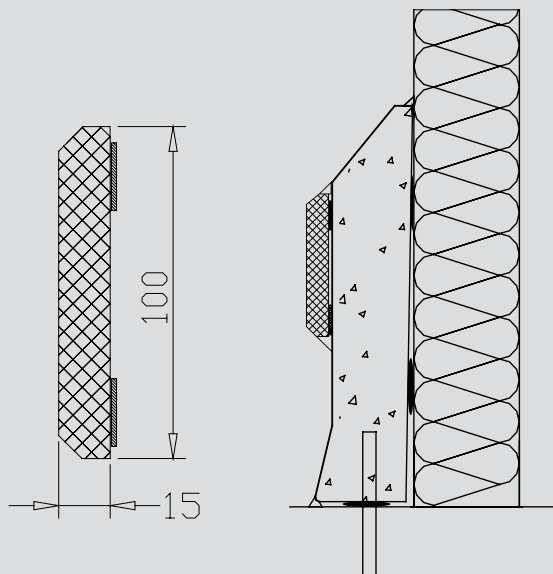
PolySto OP30F на плиточном полу с PE защитной полосой.
