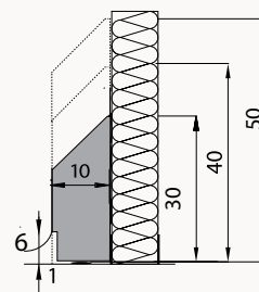
IP 30-40-50 С ВЫКРУЖКОЙ / ПРЯМОЙ
