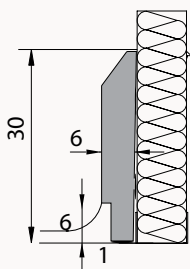
OP30RB CLEANROOM С ВЫКРУЖКОЙ
