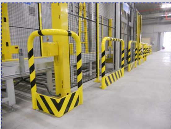
PolySto PMA (kairėje) ir PML (dešinėje) montuojama ant betoninių grindų.
