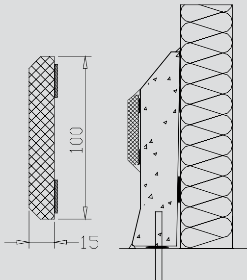
PolySto OP30F įrengta ant plytelėmis dengtos grindų dangos, atlaikantis ekstremalius poveikius (Selfadhesive- savaime prilimpantis).
