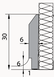
OP30RB CLEAN ROOM SU VIDINIŲ ĮGILINIMU
