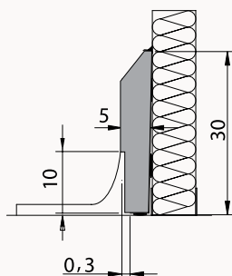
OP30RB CLEAN ROOM SU VIDINIŲ ĮGILINIMU
