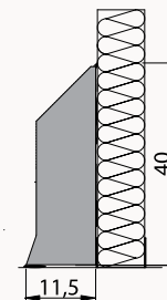
IP 30-40-50 SU VIDINIŲ ĮGILINIMU ARBA TIESUS
