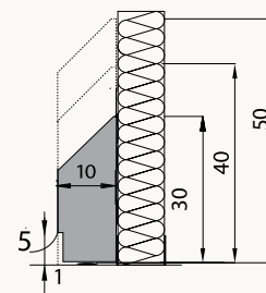
IP 30-40-50 SU VIDINIŲ ĮGILINIMU ARBA TIESUS
